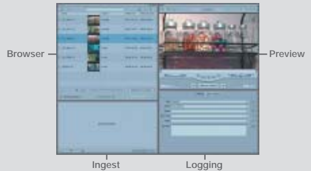
Ingest
