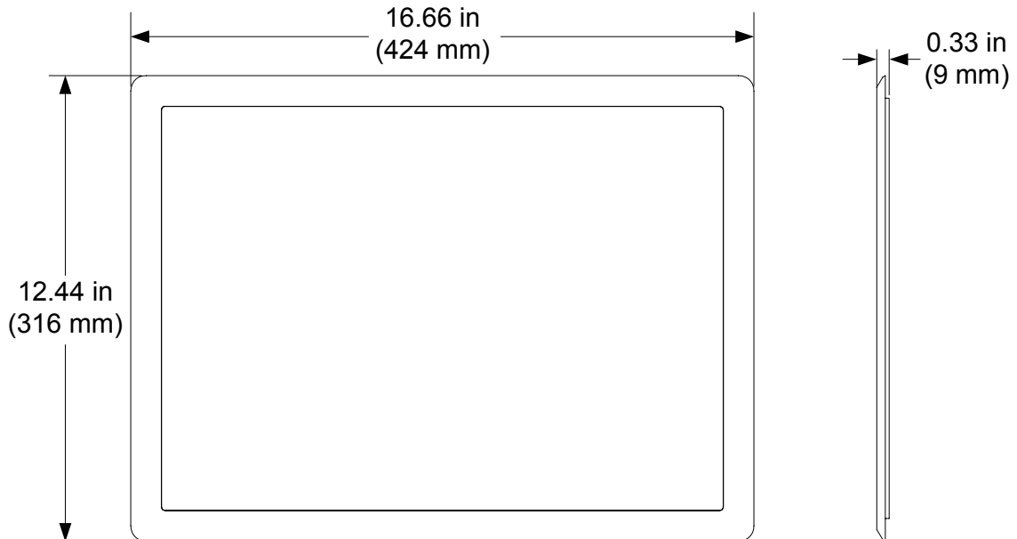
Overall Dimensions (Bezel)
