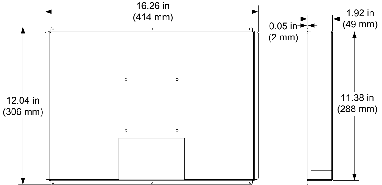
Overall Dimensions (Bezel)
